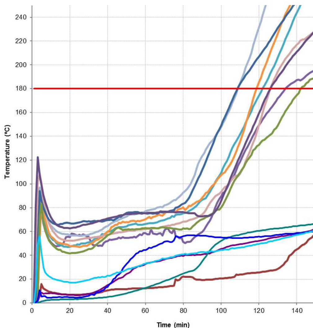
Graphique 16 : Températures maximales de l'échantillon 7.
