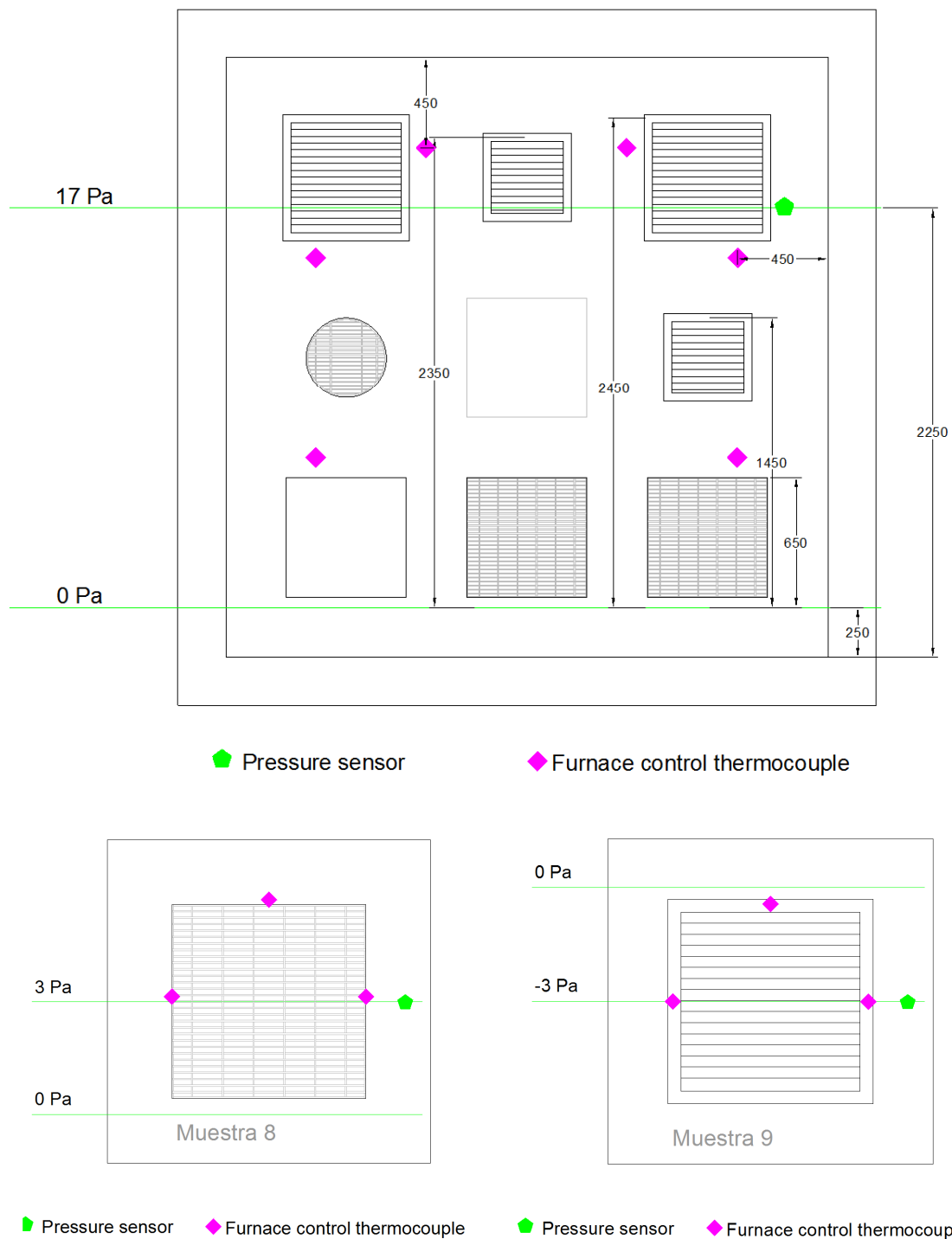
Figure 1 – Position des équipements de mesure et de pression du four.
